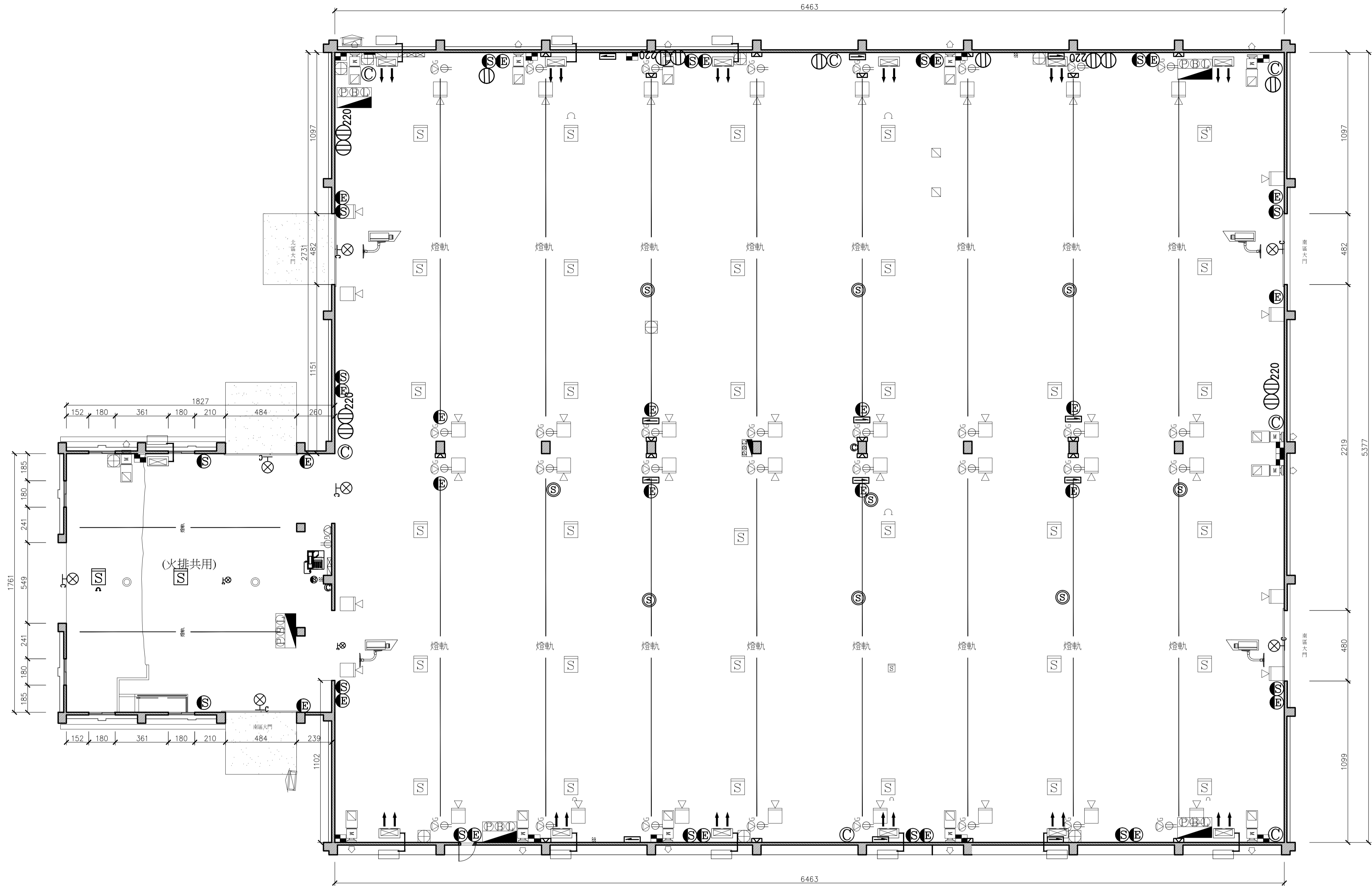
15.16號倉庫平面圖
