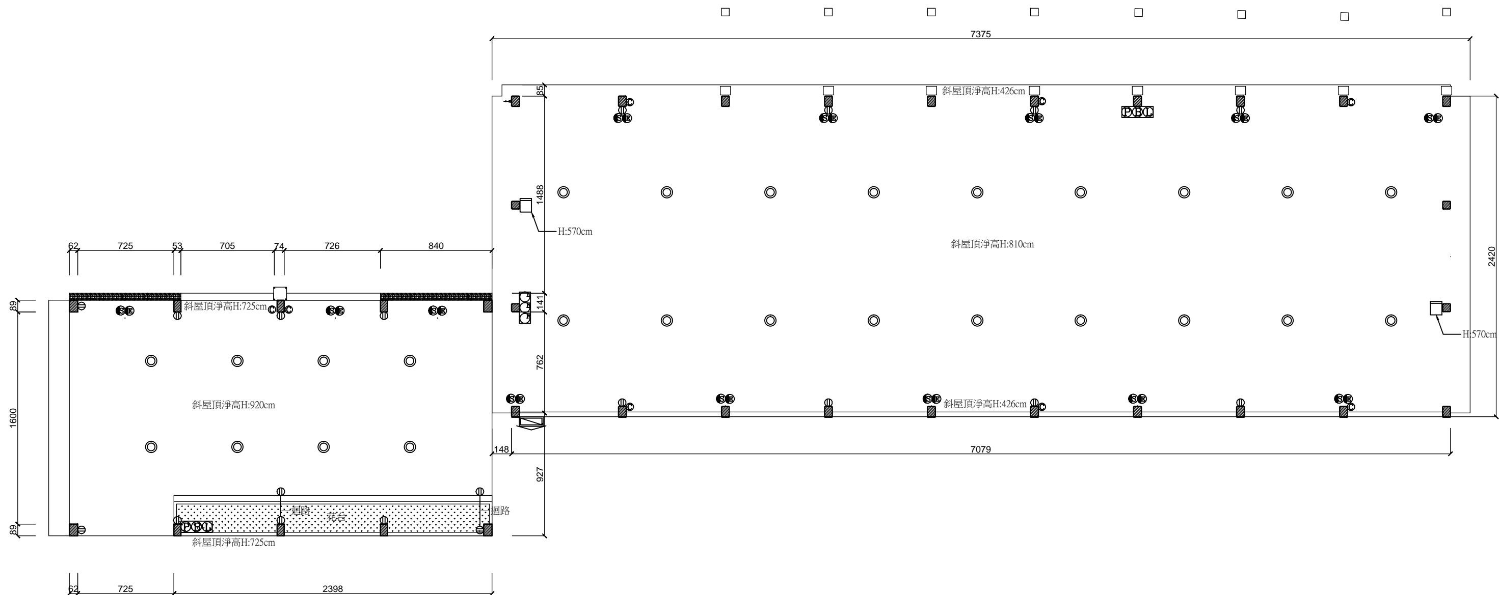
N 7號、8號倉庫平面圖
